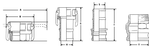
Tipo C Raccordo con portagomma serrato FED MIL
